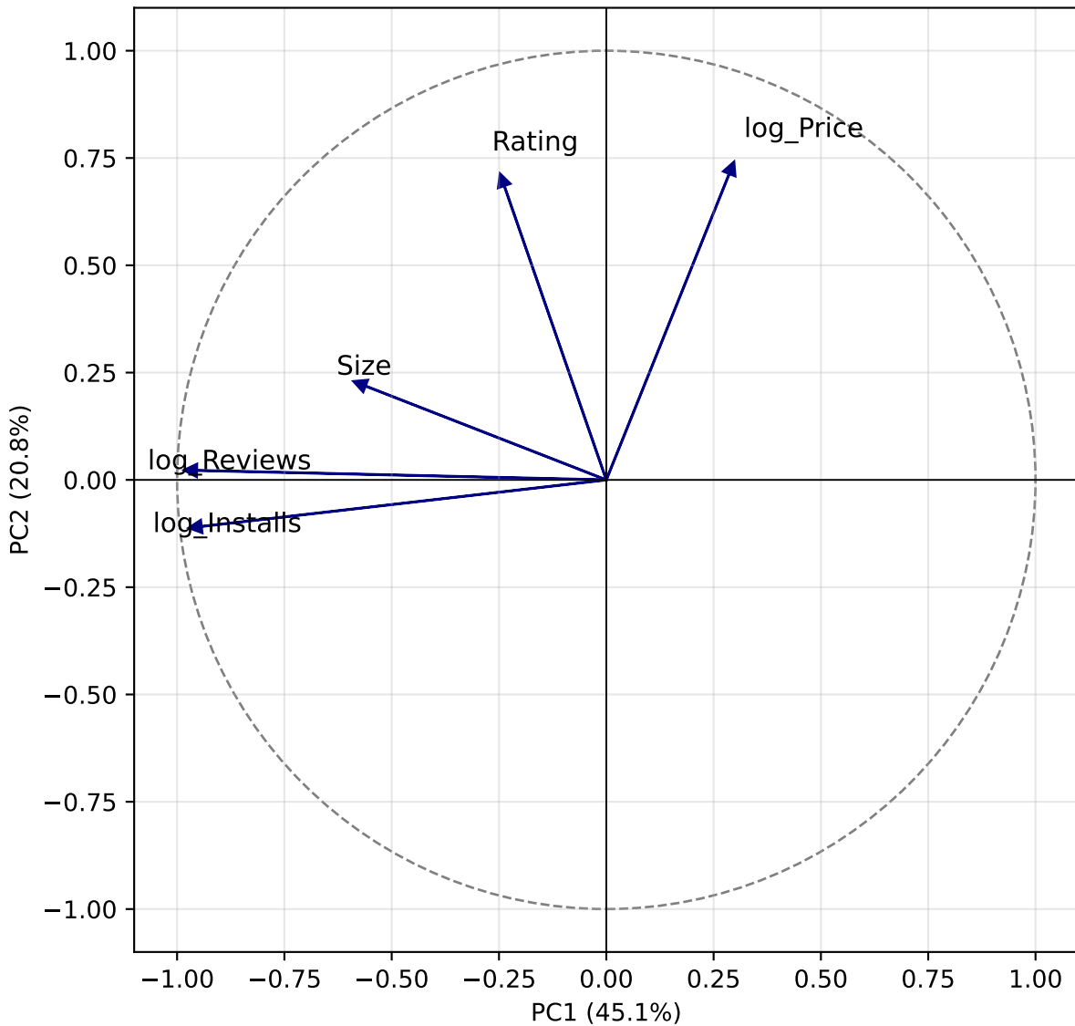
PCA Correlation Circle
