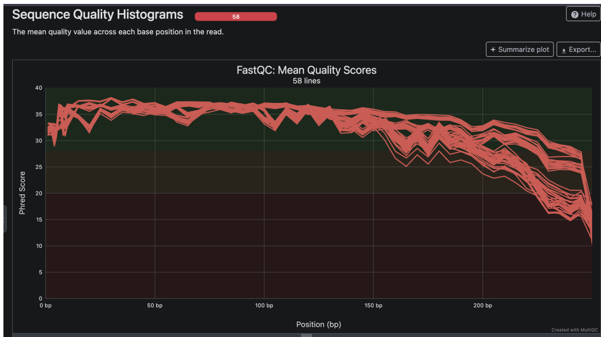
Рис. 2: Качество прочтений по позициям (Sequence Quality Histograms), все 58 файлов.
