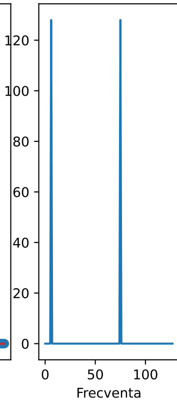
Numpy FFT
