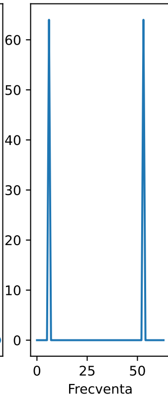
Numpy FFT
