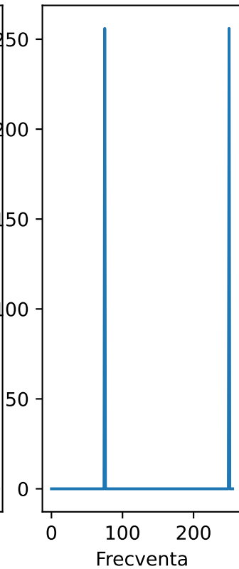
Numpy FFT
