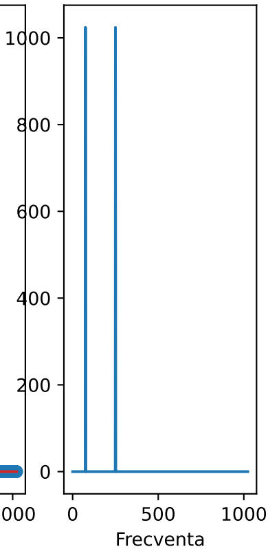
Numpy FFT
