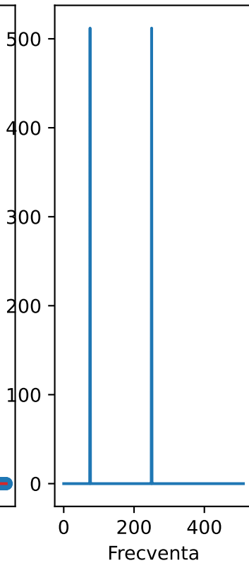
Numpy FFT
