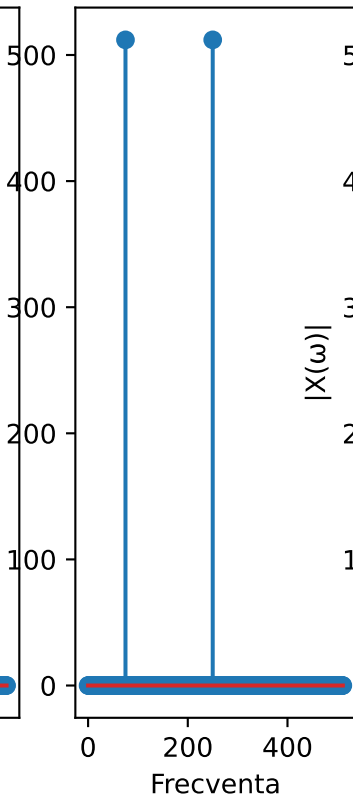
FFT
