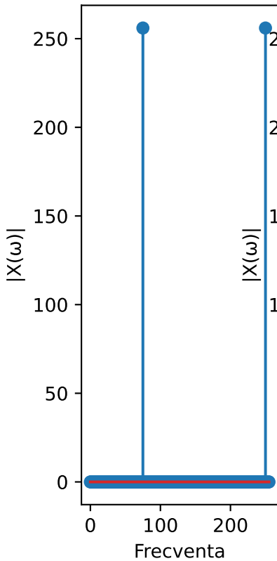
DFT
