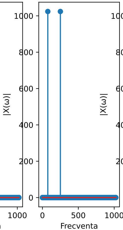
FFT
