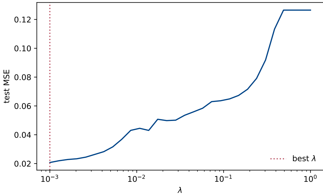
Lasso, degree 10
