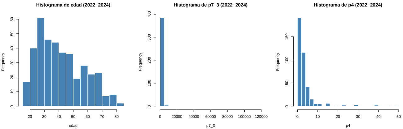
Gráficas 1, 2, 3. Histogramas de las variables edad, p7_3 (Gasto en libros) y p4 (Libros leídos) para el periodo 2022-2024.
