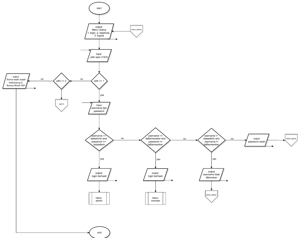
Gambar 1.1 Flowchart pada menu login dan logout
