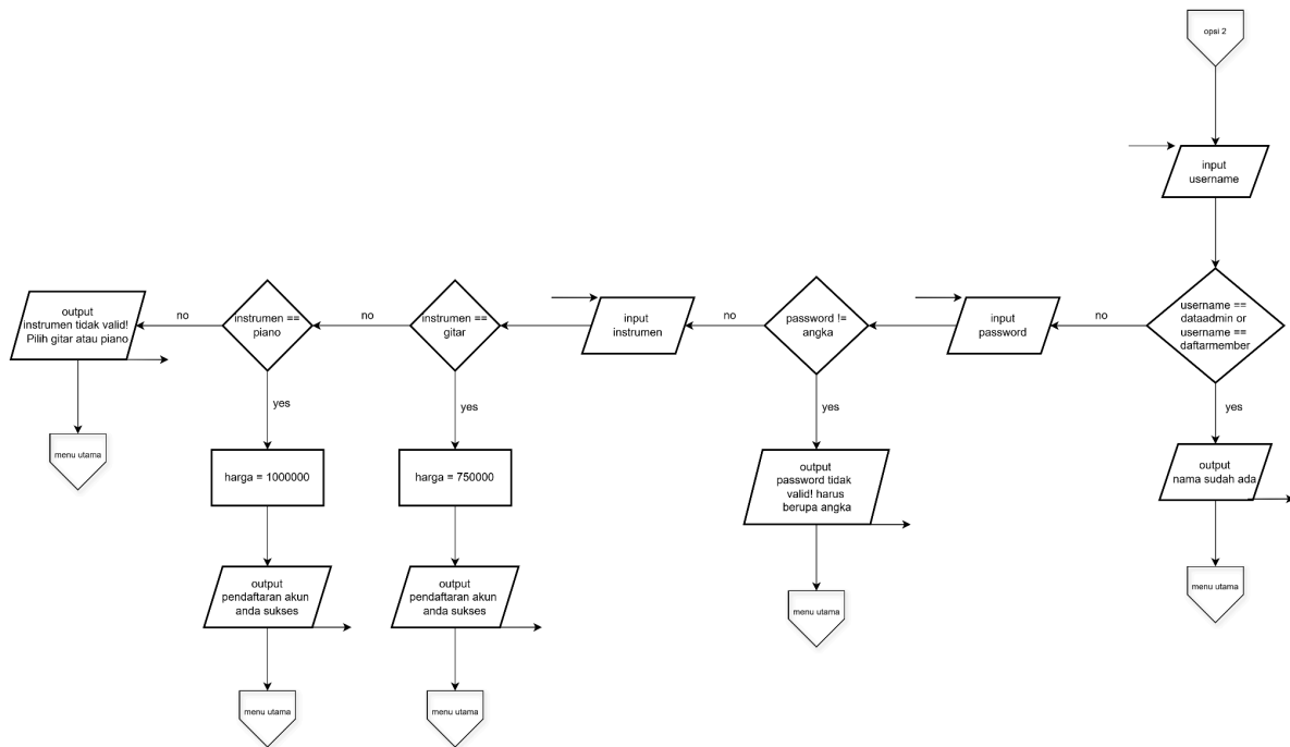
Gambar 1.2 Flowchart pada menu registrasi
