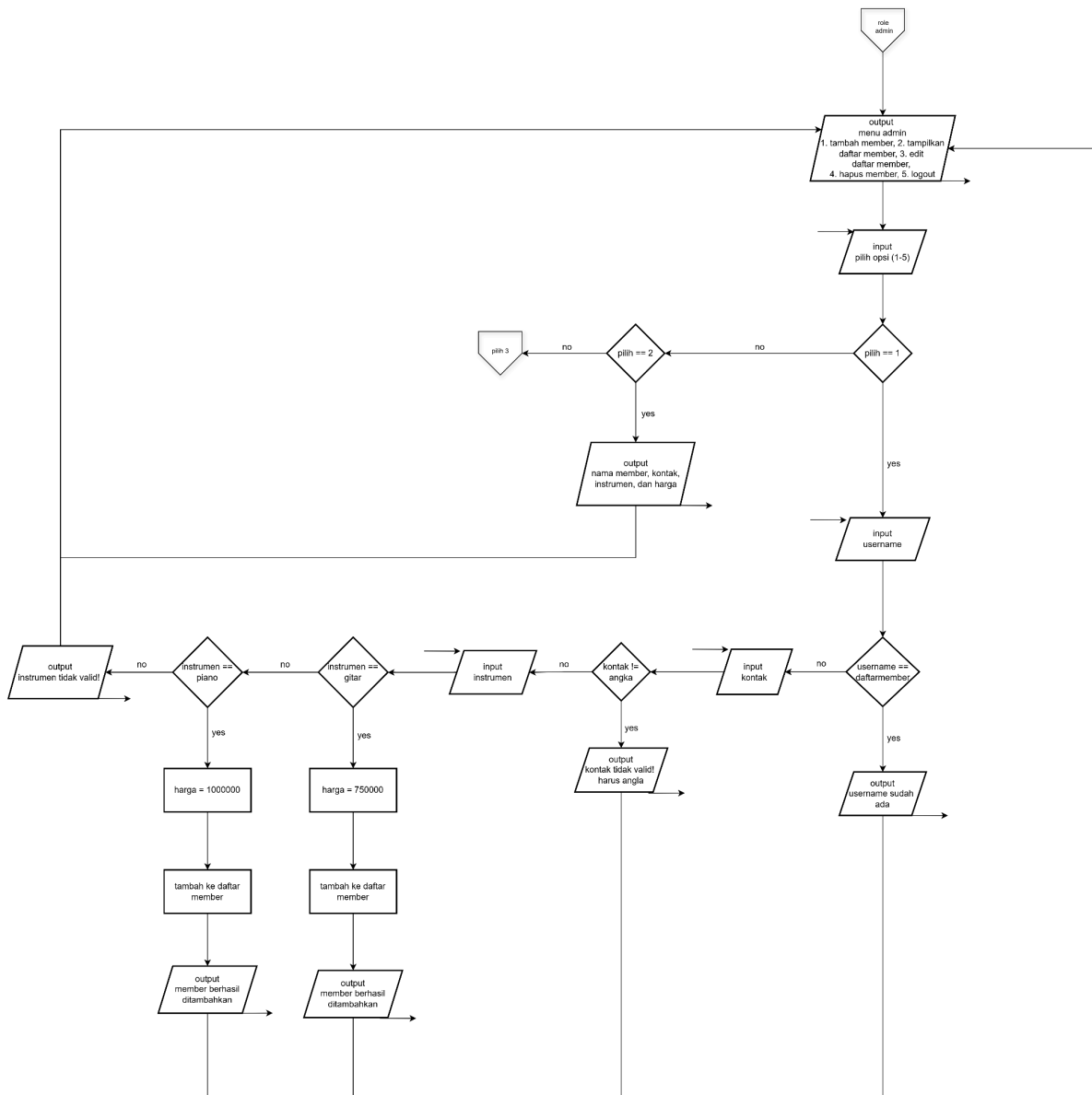
Gambar 1.3 Flowchart pada menu admin opsi 1 dan 2
