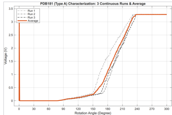
แสดงค่าที่ได้จากการเก็บผลการทดลอง Rotary Potentionmeter Series A
