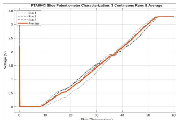
แสดงค่าที่ได้จากการเก็บผลการทดลอง linear Potentiometer Series B
