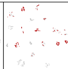
DP3
