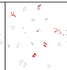
\pi_0
