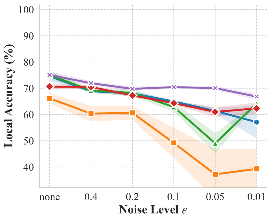
Oxford_Flowers
