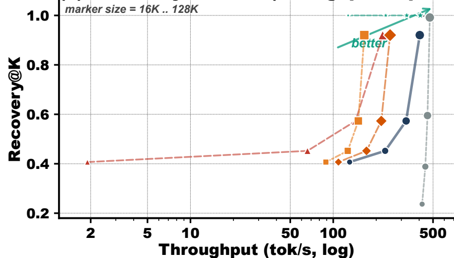
(d) Efficiency frontier (throughput × quality)
