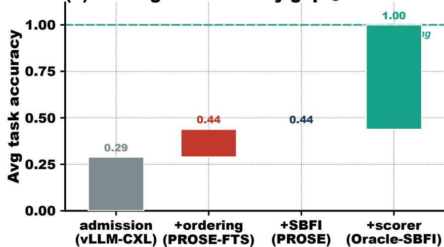
(d) Closing the accuracy gap @ 128K
