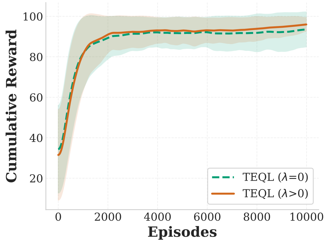
Pendulum
