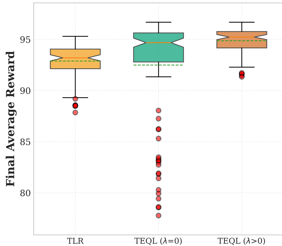
Pendulum
