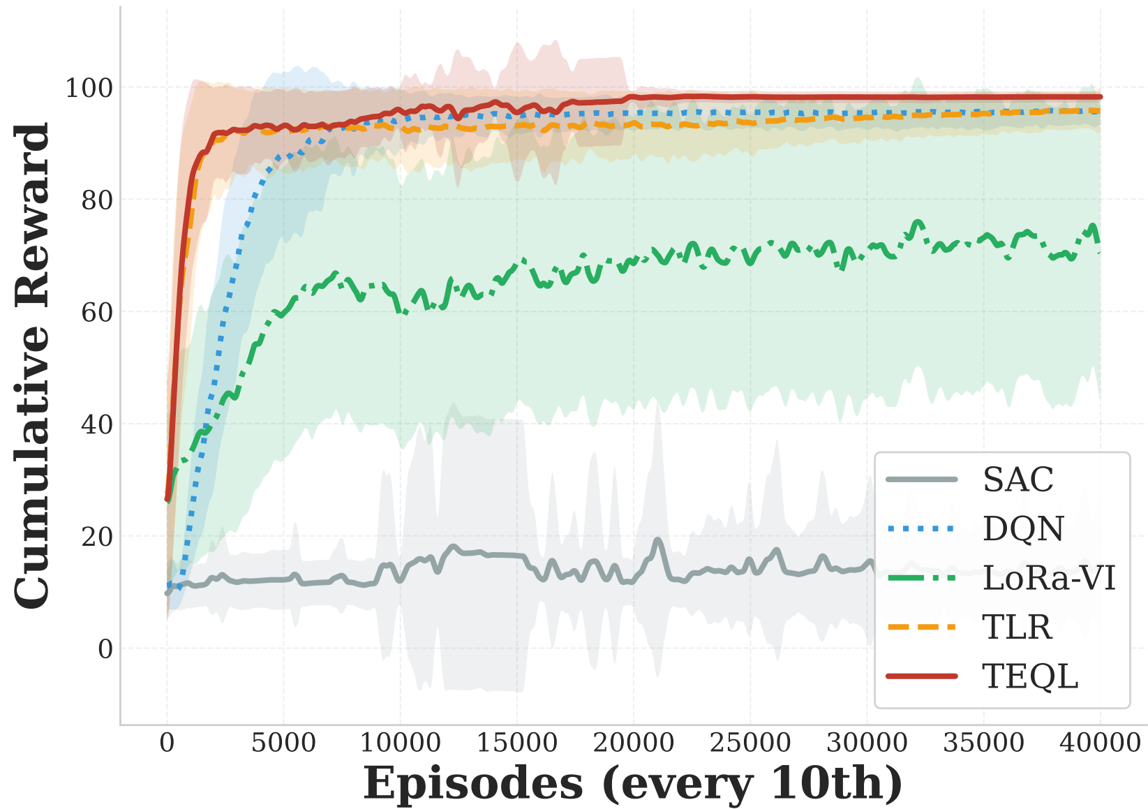
Pendulum
