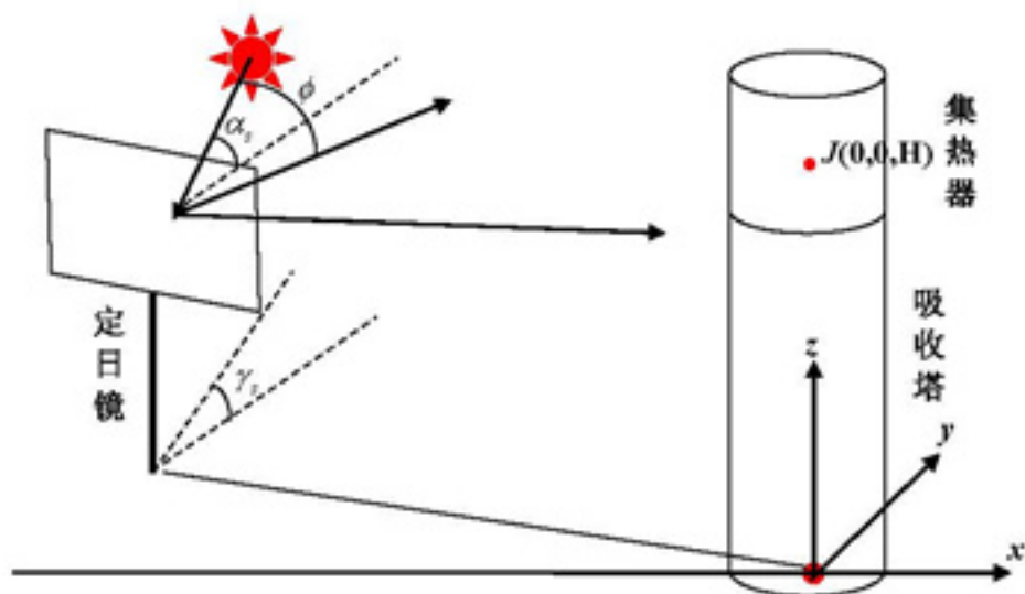
图 1：定日镜场的大地坐标系
