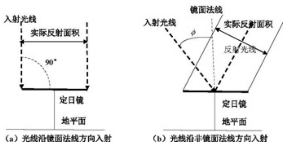
图 8：余弦损失的示意图
