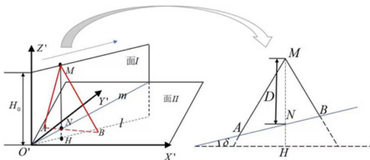
图 13: 三维空间到二维空间的转化
