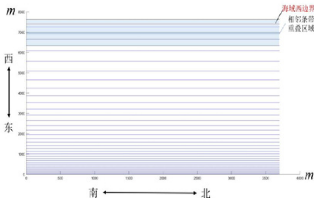
图 18: 最优测线布设
