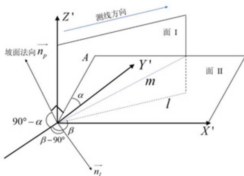
图 11: 问题二几何关系分析
