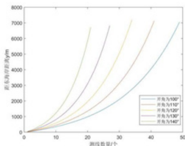
图 19: 开角灵敏度分析
