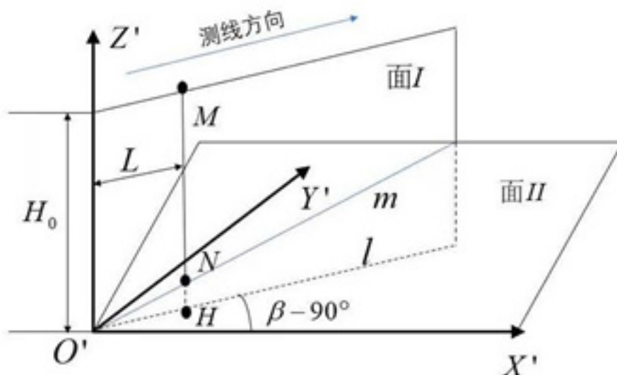
图 12: 海水深度计算
