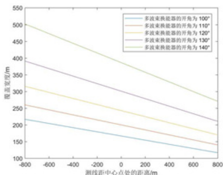
图 6: 覆盖宽度随开角的变化
