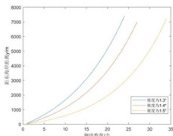
图 20: 坡度灵敏度分析
