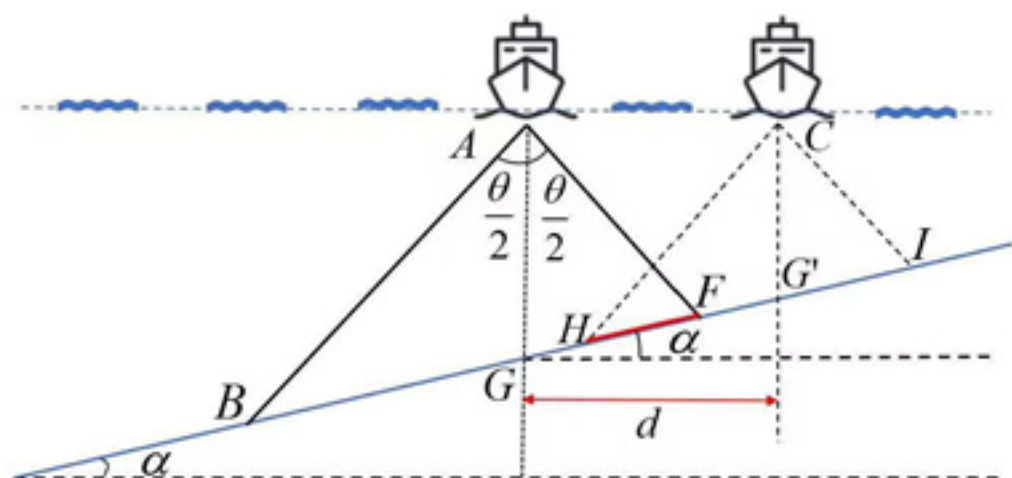
图 5: 相邻条带之间的重叠
