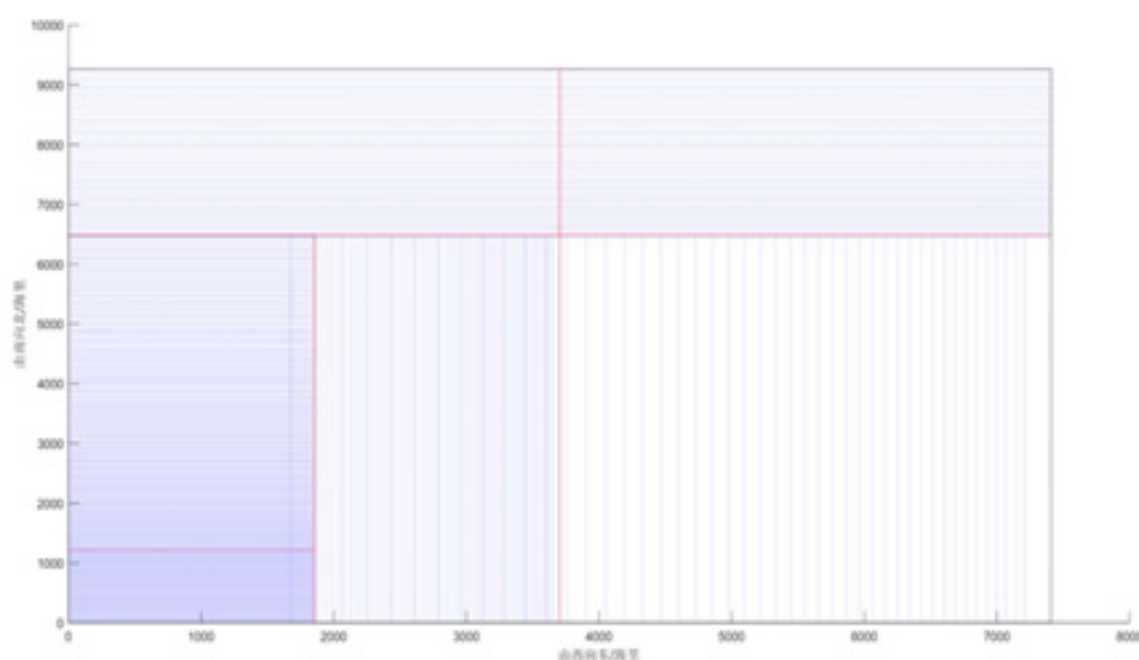
图 26: 多波束测线布置
