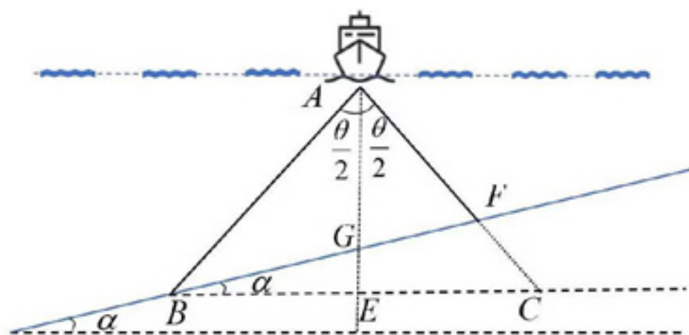
图 4：覆盖宽度计算
