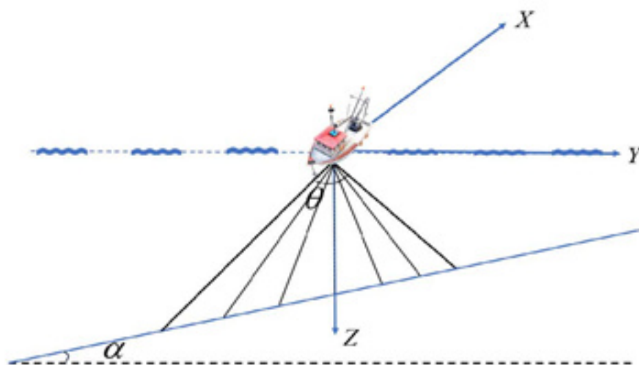
图 2：多波束测量坐标系的建立
