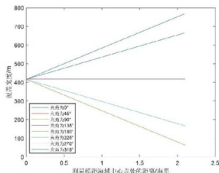
图 14: 不同 \beta 角对覆盖宽度的影响
