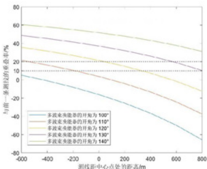
图 7: 重叠率随开角的变化
