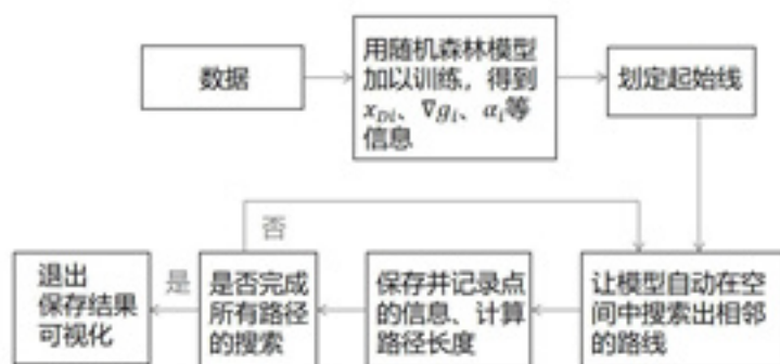
图 21 航线计算流程图示
