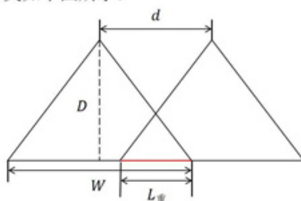
图 1 水平状态下重叠率的定义
