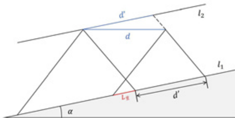
图 3 投影测线间距
