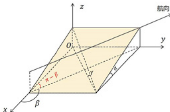
图 8 \beta = 135^\circ 时几何关系图
