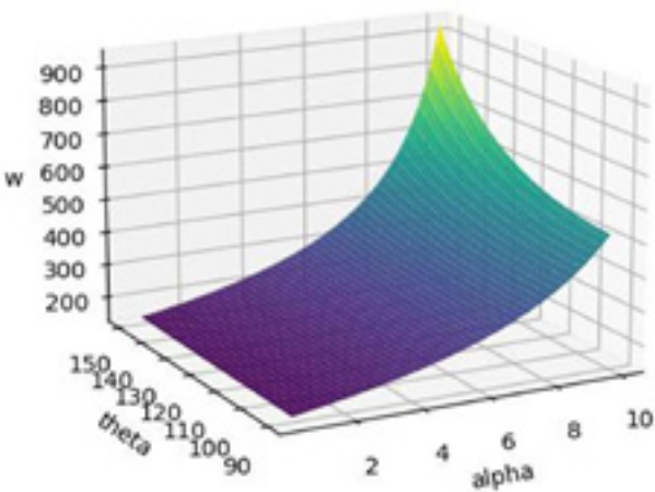
图 18 不同张角和坡度下最大覆宽变化图
