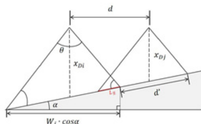
图 5 投影位置简图
