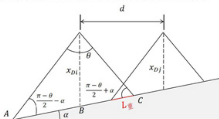
图 4 相关位置简图
