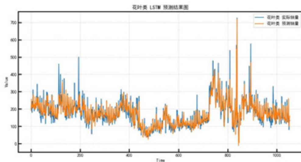
图 21 花叶类 LSTM
