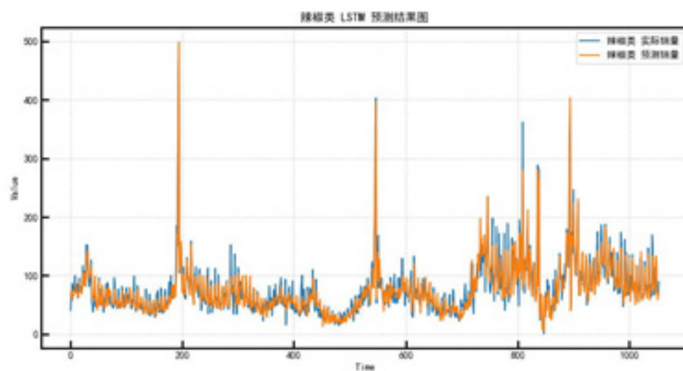
图 25 辣椒类 LSTM
