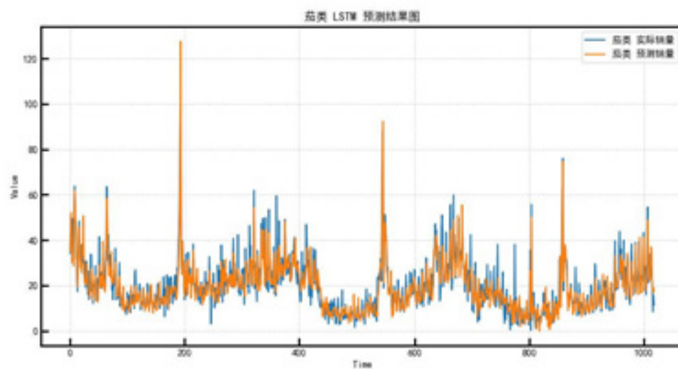
图 24 茄类 LSTM
