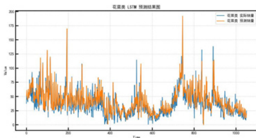
图 22 花菜类 LSTM
