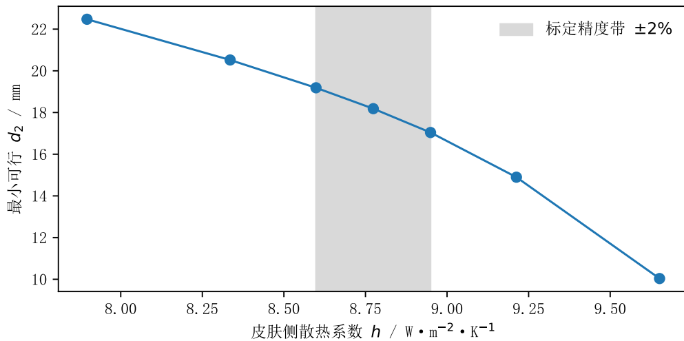
图 3 问题二最小可行厚度对皮肤侧散热系数的依赖
