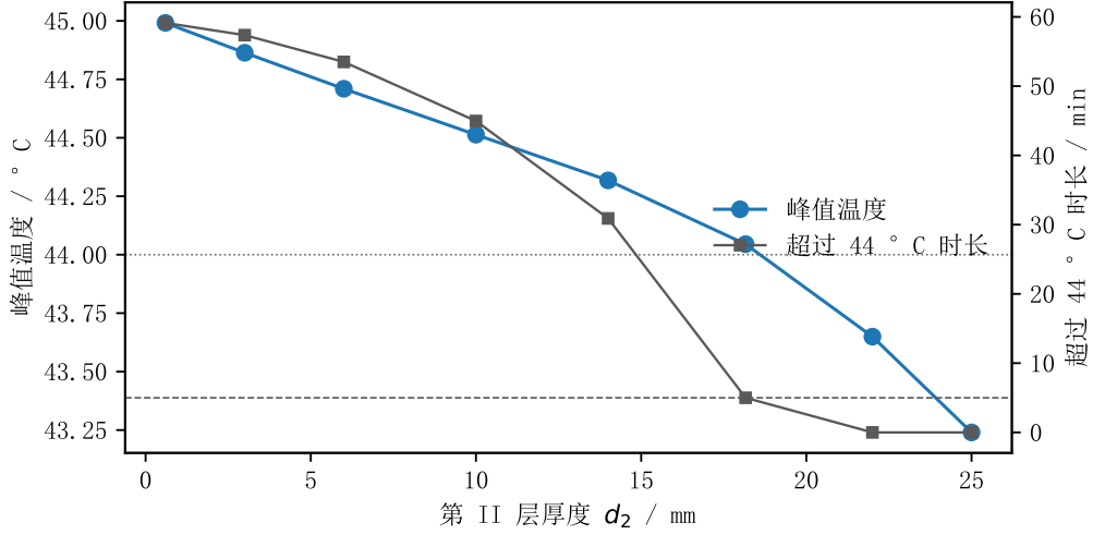
图 2 第 II 层厚度对峰值温度与越阈时长的影响
