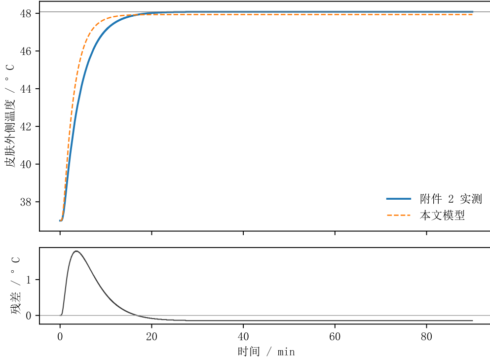
图 1 皮肤外侧温度：模型与附件 2 实测对比及残差
