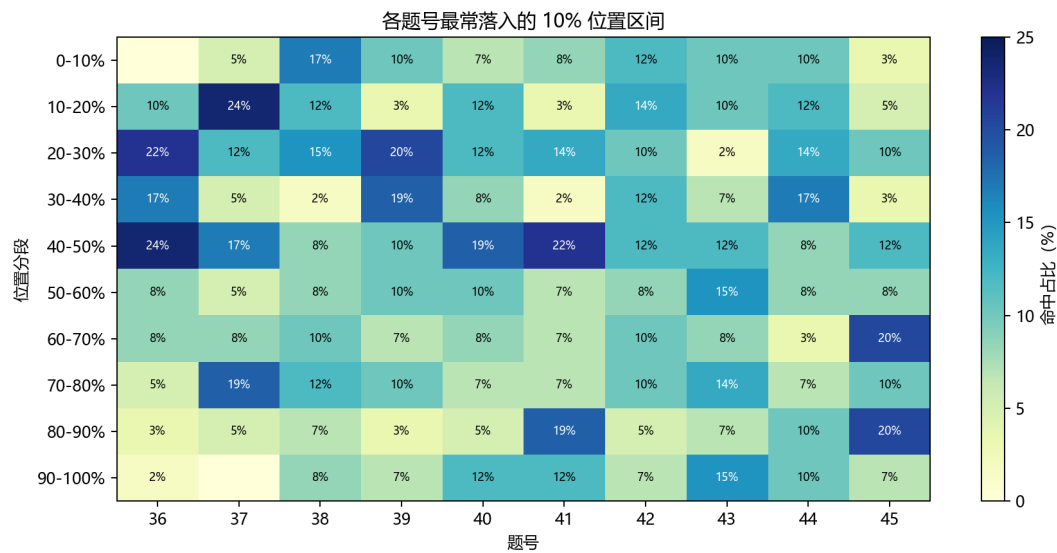
图 3: question_position_band_heatmap.png
