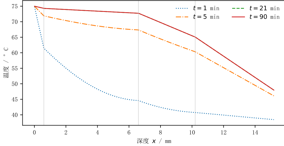
图2 四层内的温度剖面随时间演化，竖线为层界
