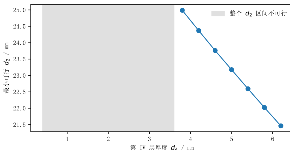
图 4 问题三前沿与不可行带
