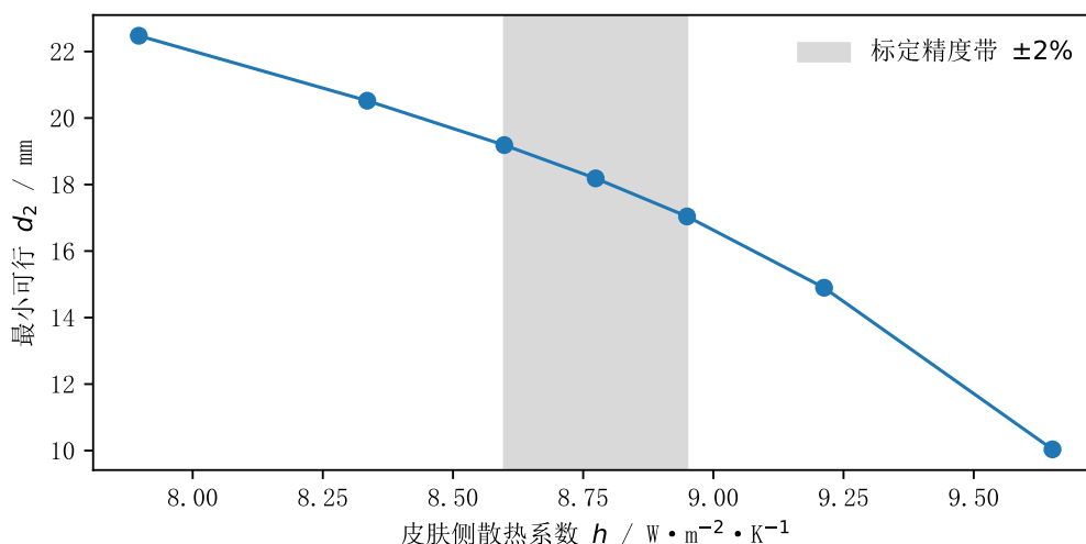
图 5 问题二最小可行厚度对皮肤侧散热系数的依赖
