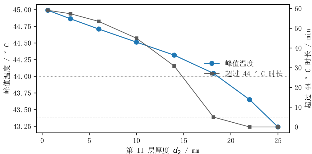
图 3 第 II 层厚度对峰值温度与越阈时长的影响
