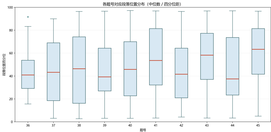
图 1: question_position_boxplot.png
