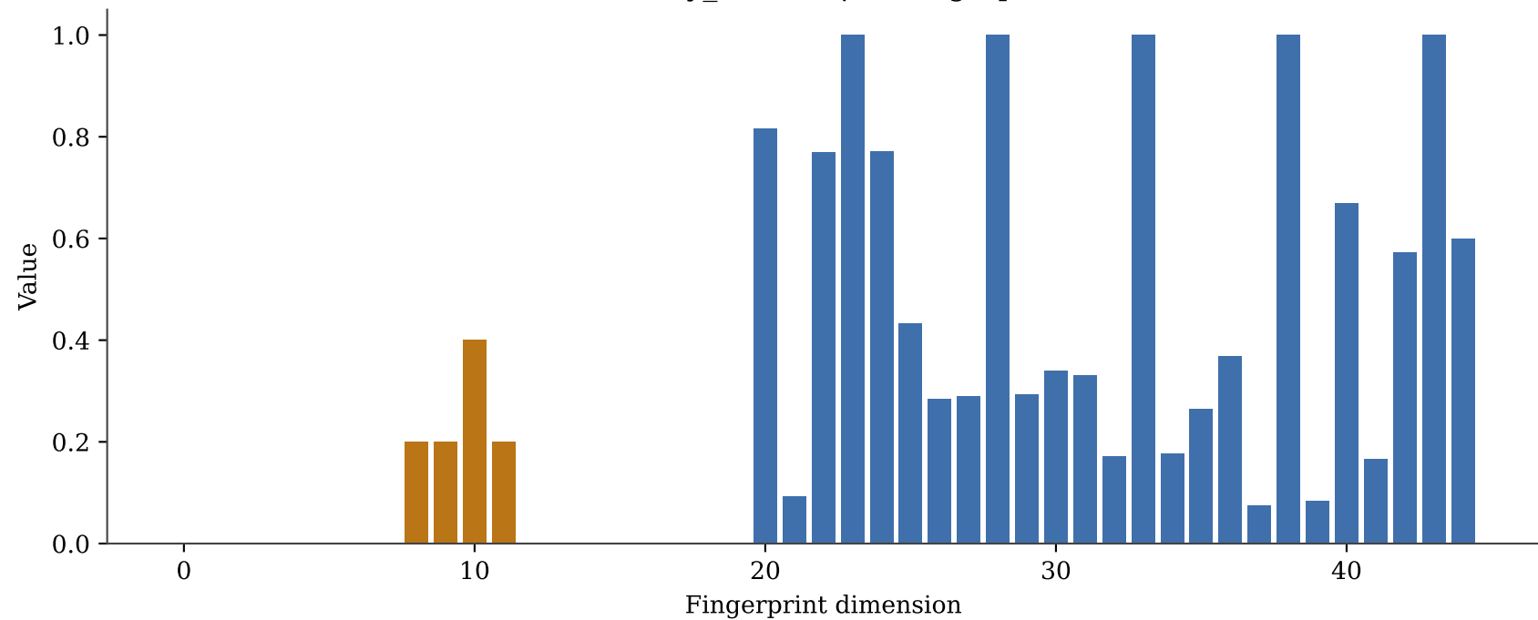
distribuidora-delivery_click — \phi(G) fingerprint [PHISHING]
