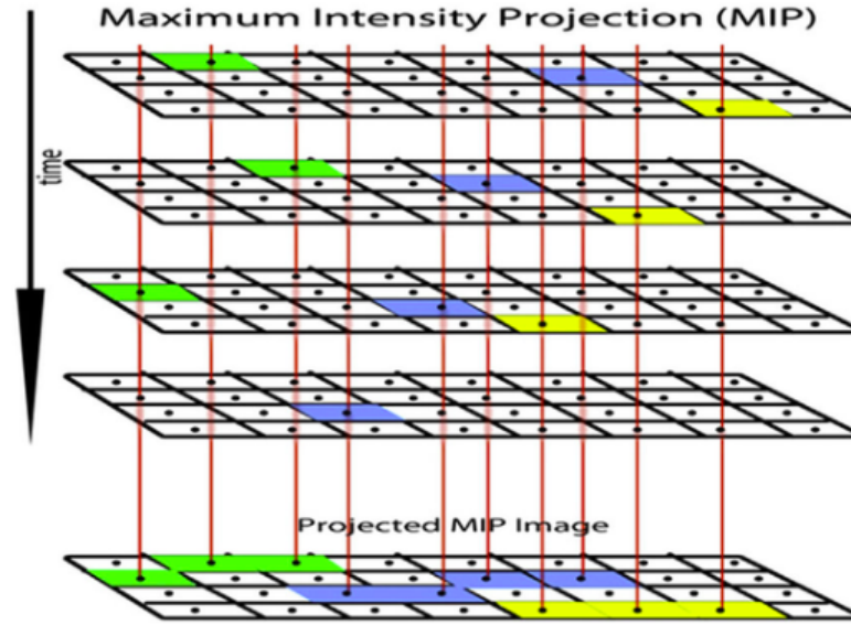
Hình 2.2: Minh họa thuật toán MIP trong trích xuất mạng lưới mạch máu từ khối dữ liệu 3D
