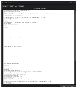
Рис. 4: Настройка интерфейсов коммутатора provider-sw-1
