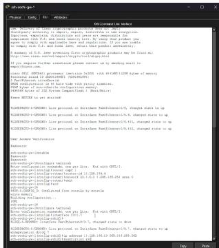
Рис. 7: Настройка маршрутизатора sch-sochi-gw-1
