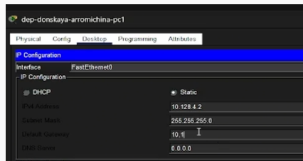
Рис. 19: Настройка IP адреса dep-pc-1
