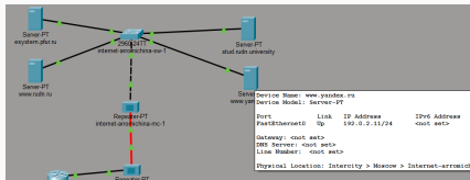
Рис. 1: Вносим изменения в схемы L2 и L3 сети, указав адреса и VLAN сети провайдера и модельной сети Интернета. Скорректируем таблицы распределения IP-адресов и портов
