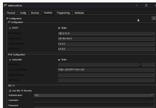
Рис. 5: Пропишем IP-адреса серверам
