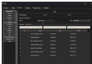
Рис. 6: Пропишем сведения о серверах на DNS-сервере сети «Донская»
