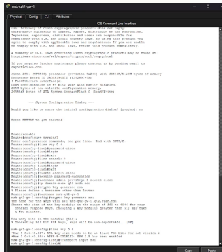
Рис. 6: Первоначальная настройка маршрутизатора msk-q42-gw-1
