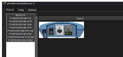
Рис. 1: На медиаконвертерах заменим имеющиеся модули на PT-REPEATER-NM-1FFE и PT-REPEATER-NM-1CFE для подключения витой пары по технологии Fast Ethernet и оптоволокна соответственно
