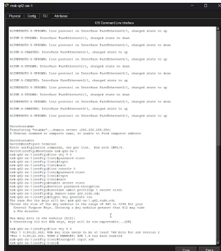
Рис. 7: Первоначальная настройка коммутатора msk-q42-sw-1
