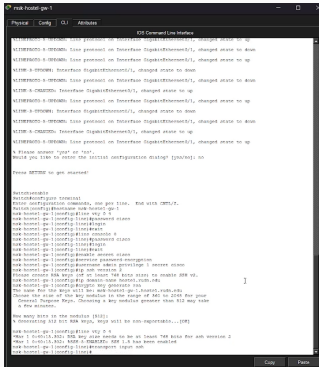
Рис. 8: Первоначальная настройка маршрутизирующего коммутатора msk-hostel-gw-1
