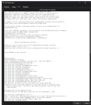
Рис. 11: Первоначальная настройка маршрутизатора sch-sochi-gw-1
