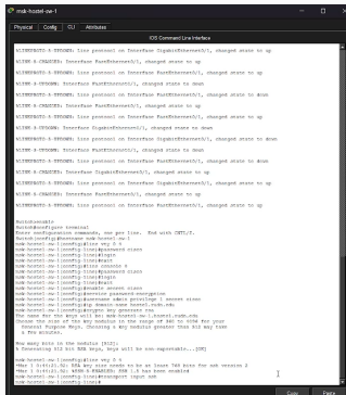
Рис. 9: Первоначальная настройка коммутатора msk-hostel-sw-1
