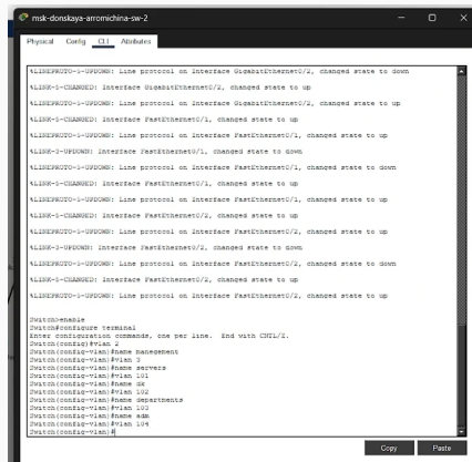
Рис. 3: Начальная настройка msk-donskaya-arromichina-sw-2
