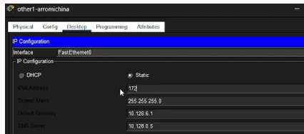
Рис. 25: Настройка other1-arromichina 172.16.0.3
