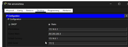
Рис. 24: Настройка file-arromichina 172.16.0.3
