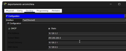
Рис. 16: Настройка deportaments-arromichina 10.128.0.0.16
