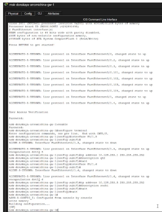
Рис. 1: Настройка интерфейсов маршрутизатора msk-donskaya-gw-1
