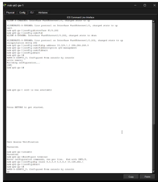
Рис. 10: Настройка маршрутизатора msk-q42-gw-1
