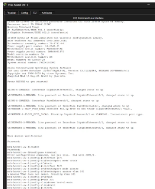
Рис. 6: Настройка интерфейсов коммутатора msk-hostel-sw-1
