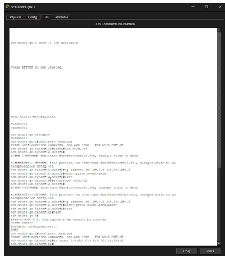
Рис. 11: Настройка маршрутизатора sch-sochi-gw-1
