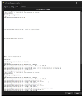
Рис. 14: Настройка NAT на маршрутизаторе msk-donskaya-gw-1
