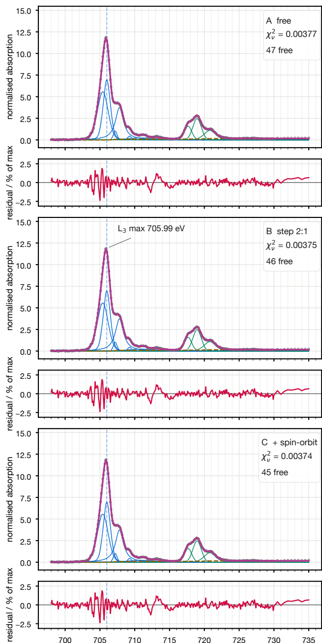
[FeCl 4 ] 2- (Fe 2+ , d 6 ) — 331 points
