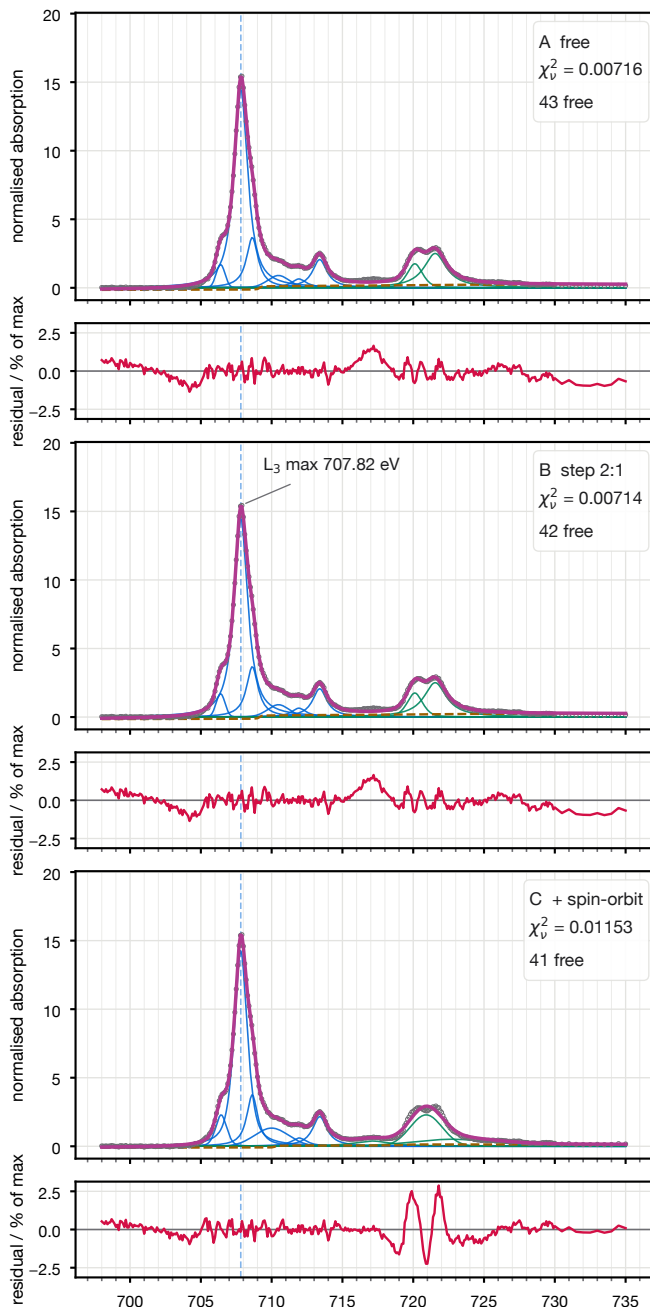
[FeCl 4 ] - (Fe 3+ , d 5 ) — 331 points
