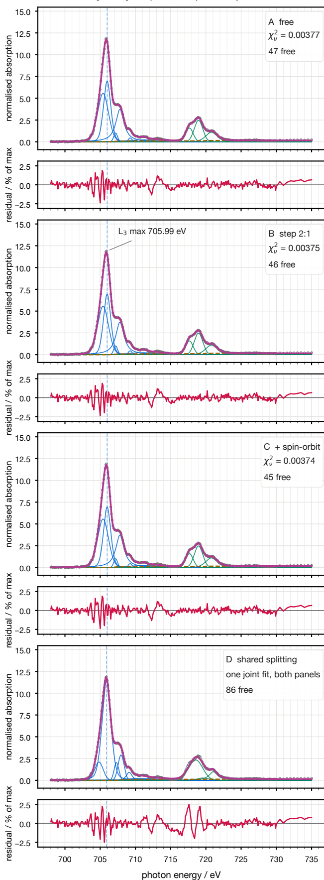
[\text{FeCl}_4]^{2-} ( \text{Fe}^{2+} , d^6 ) — 331 points
