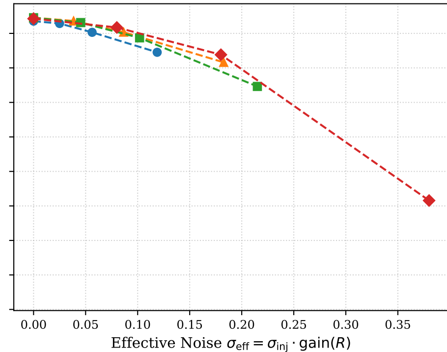
FlexiViT-B
