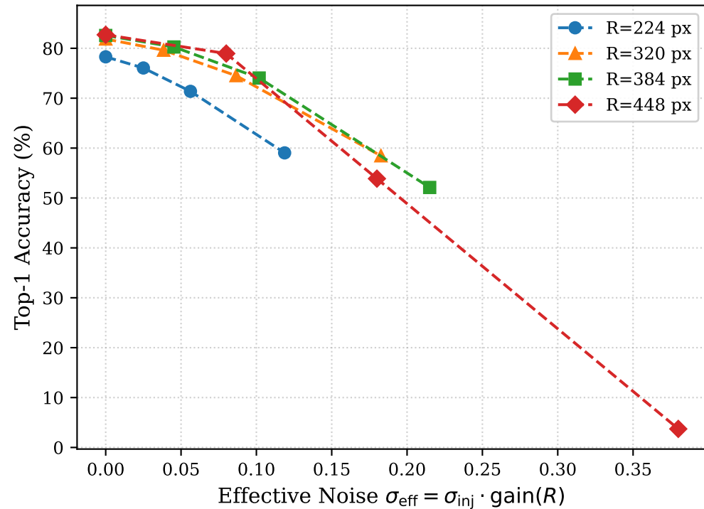
EfficientNet-B3
