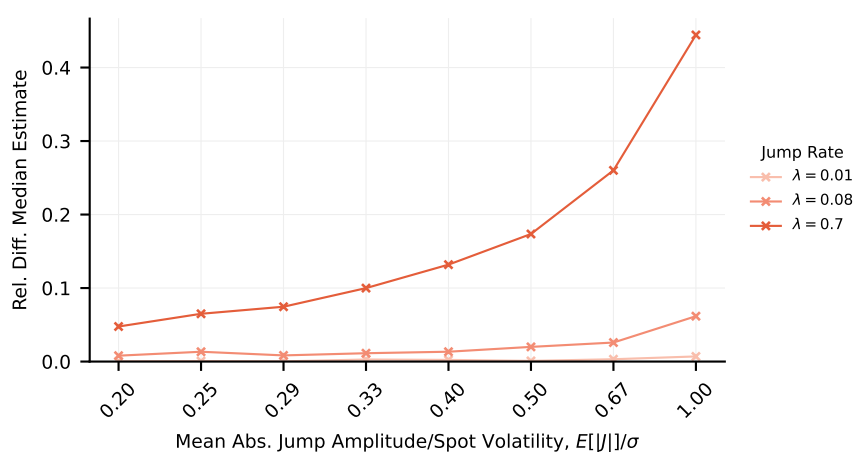
(d) Vasicek Model vs. MRJD Model, Asian Put Option, 12 observations
