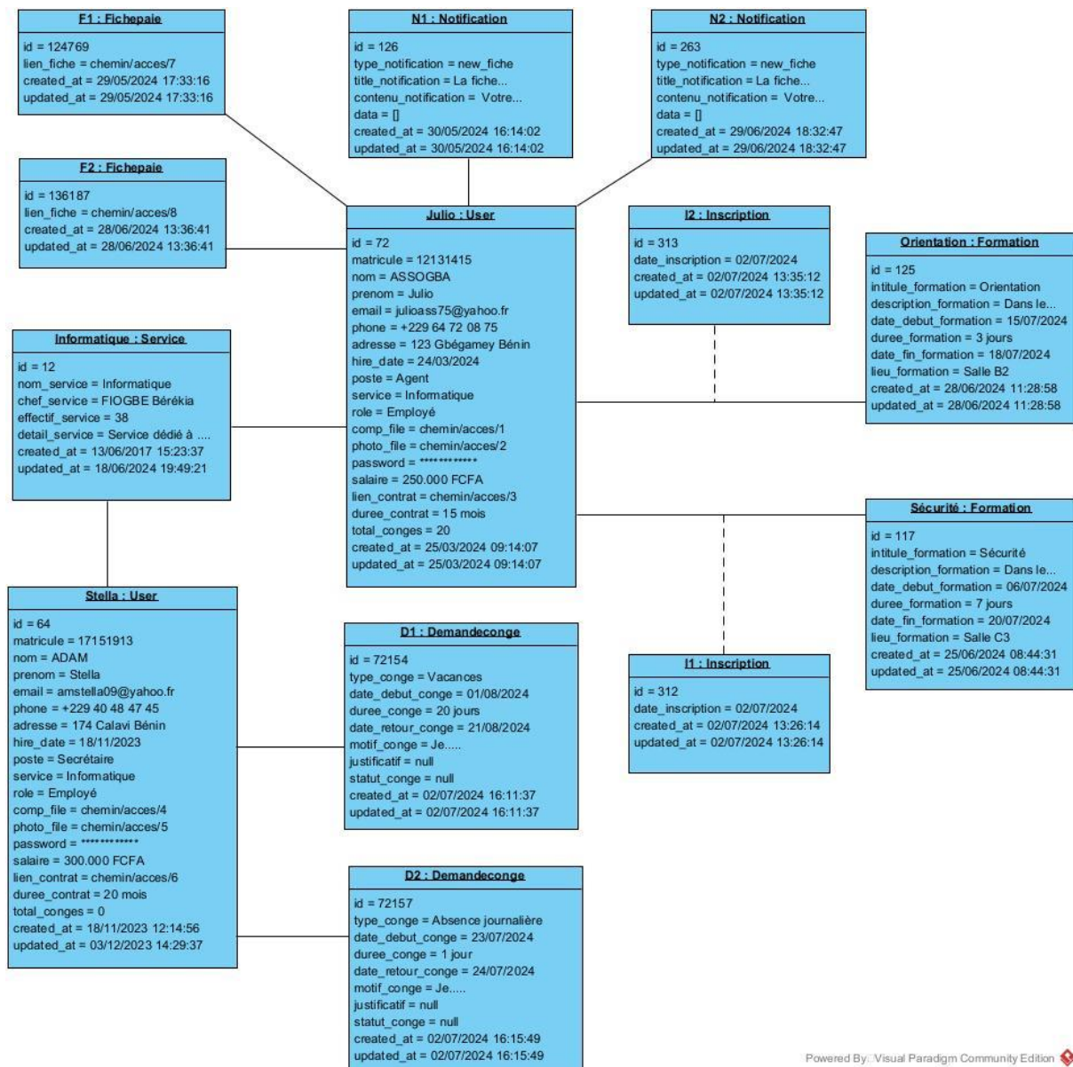
Figure4-b : Diagramme d'objets
