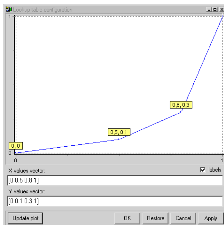
Rys. 1. Okno konfiguracyjne krzywej przetwarzania bloku Lookup table .
