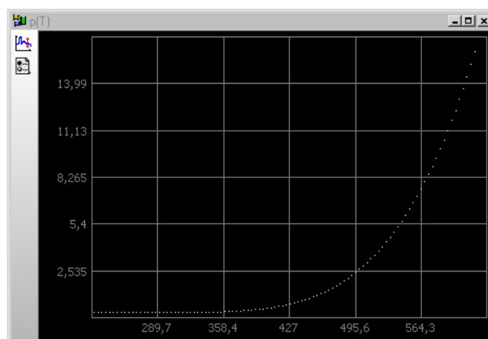
Rys. 1). Przykład zadziałania bloku Sat. steam p(T) . (konfiguracja: manual_examples.xml→Water-steam dependencies).
