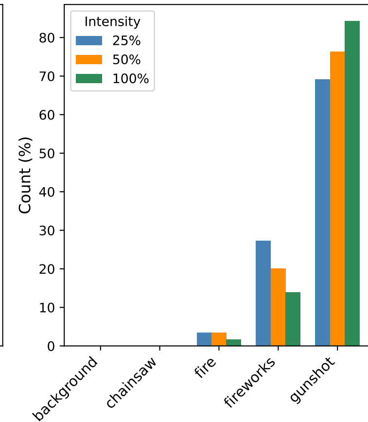
FIRE - HF
