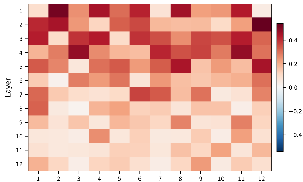
Base GPT-2
