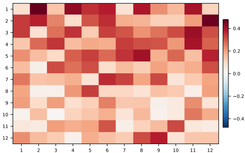
Base GPT-2
