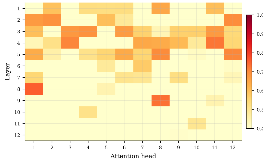
Base GPT-2
