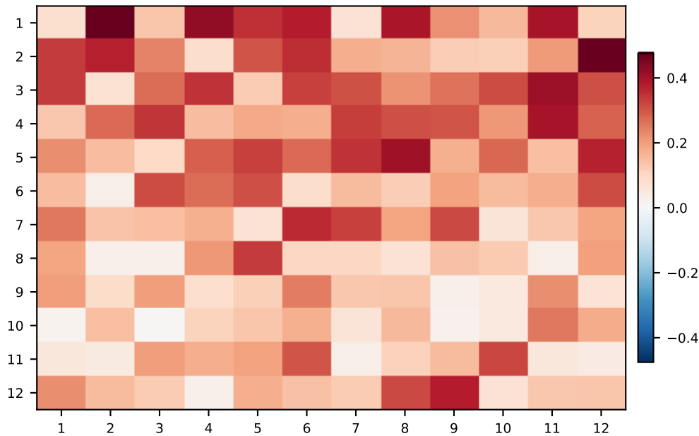
Base GPT-2
