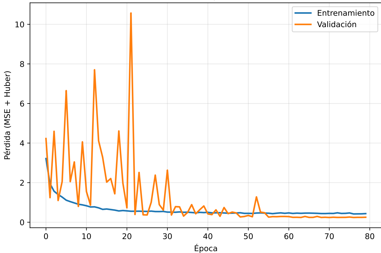
Curvas de pérdida
