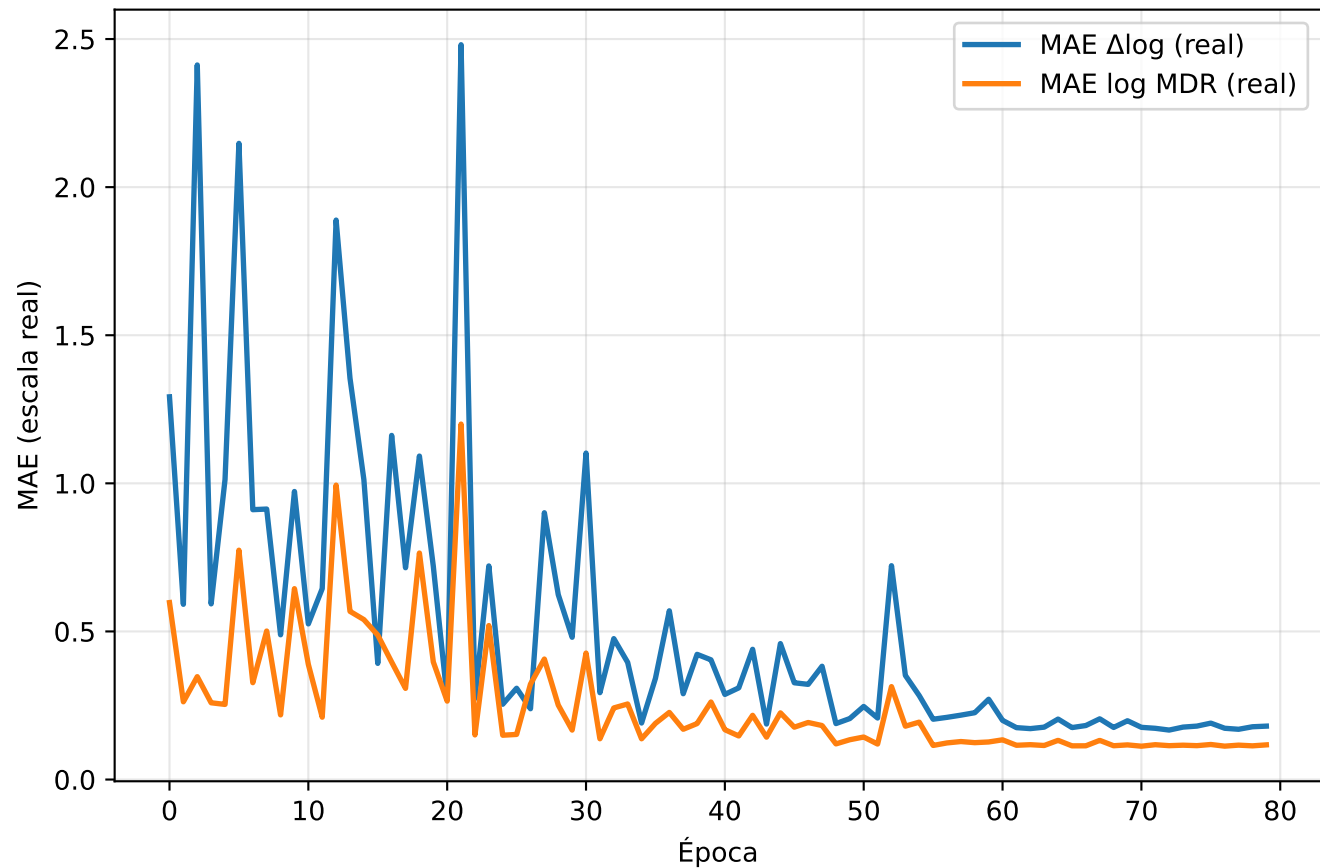
Evolución del MAE en validación
