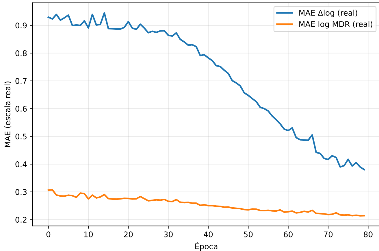
Evolución del MAE en validación - LSTM
