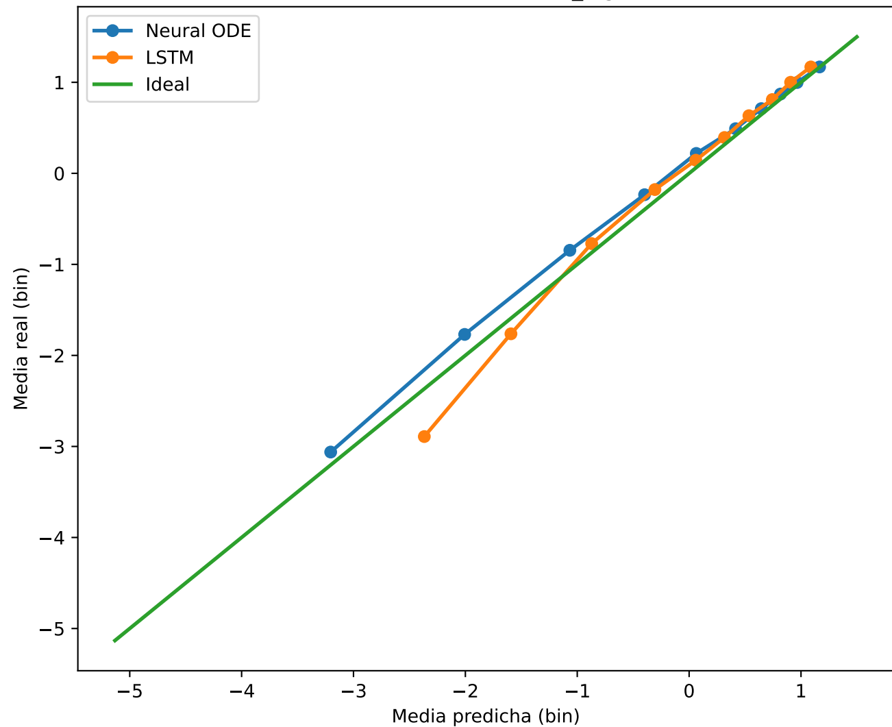
Curva de calibración: delta_log (TEST)
