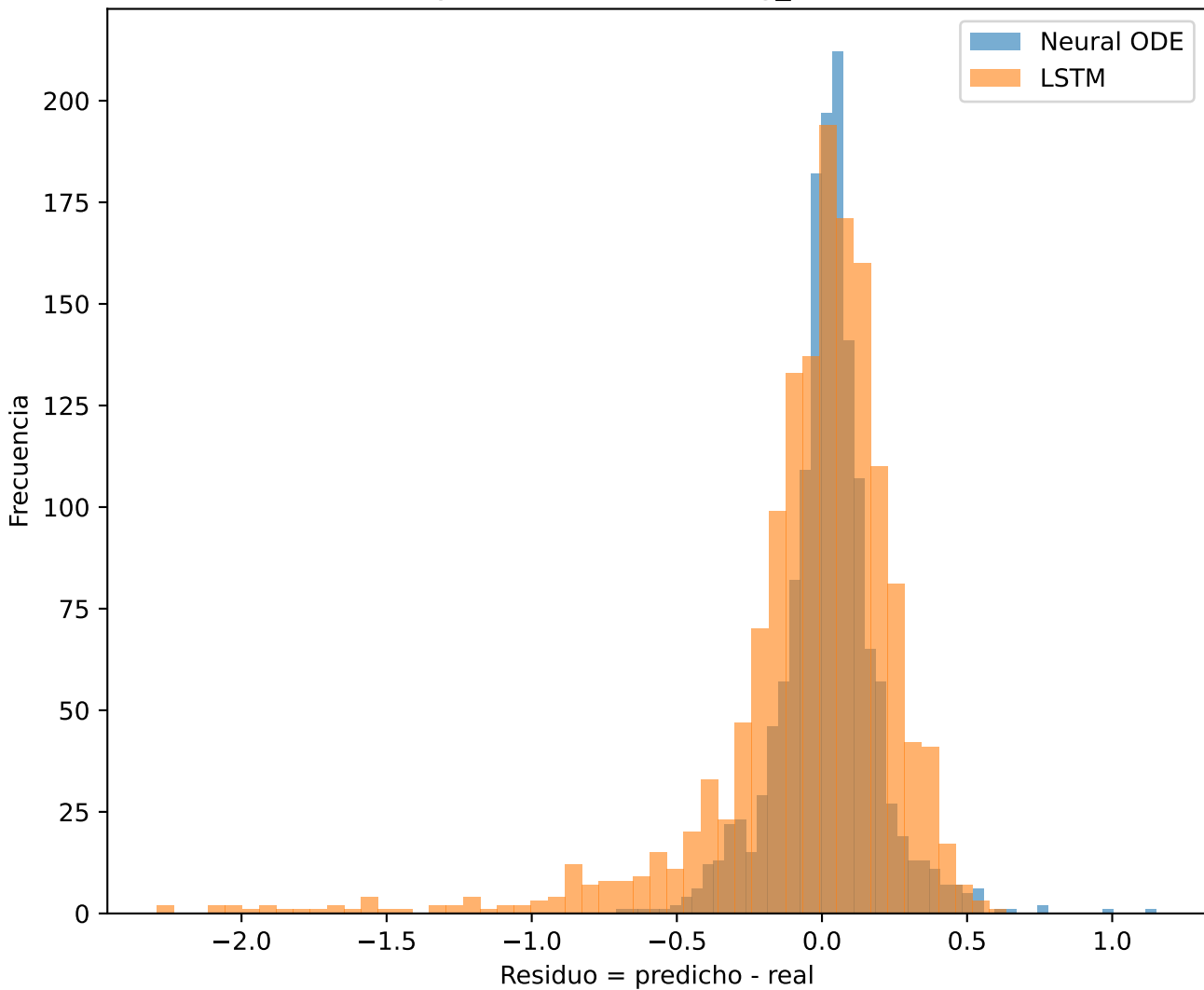
Histograma de residuos: log_mdr (TEST)
