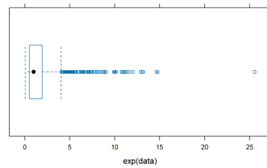
(d) Boxplot
