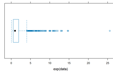
(d) Boxplot
