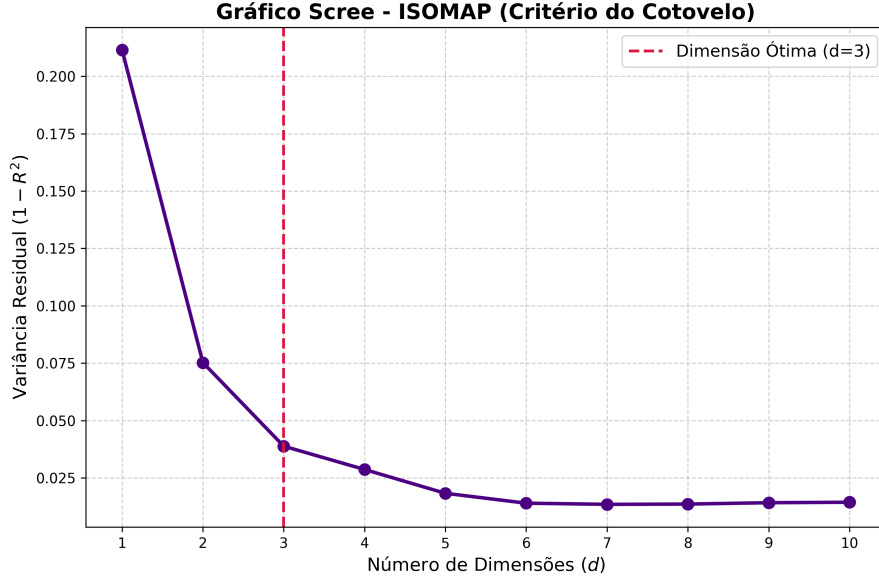
Figura 10: Redução de dimensão via Isomap para a estrutura 1OMP. A flexão abrupta no parâmetro d = 3 indica a dimensionalidade intrínseca ideal para a representação das flutuações dinâmicas da MBP.
