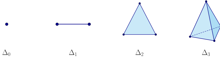
Figura 4: Representação dos simplexes: 0-Simplexo (Ponto ou vértice), 1-Simplexo (Segmento ou aresta), 2-Simplexo (Triângulo com face preenchida) e 3-Simplexo (Tetraedro preenchido).
