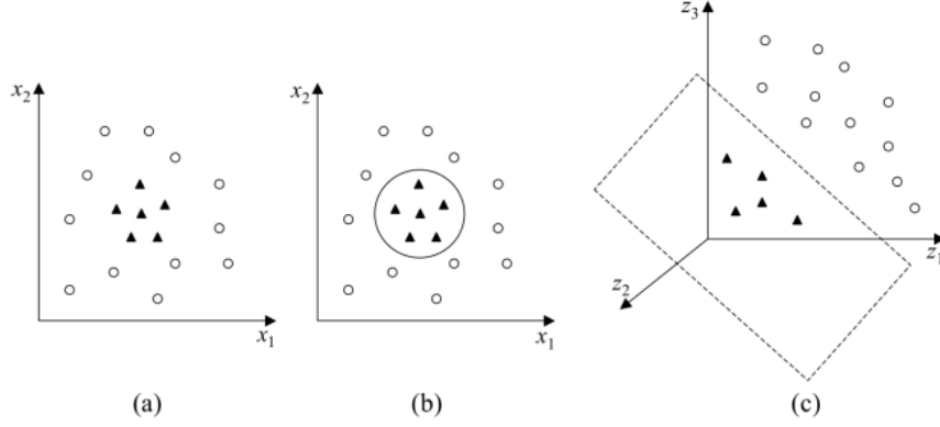
Figura 19: (a) Conjunto de dados não linear expressado em 2 dimensões; (b) Fronteira não linear no espaço de entradas; (c) Fronteira linear no espaço de características representado em 3 dimensões. Fonte: retirado de [13].
