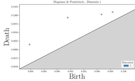
(b) Diagrama de persistência
