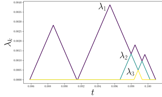
(d) Landscape (2D)
