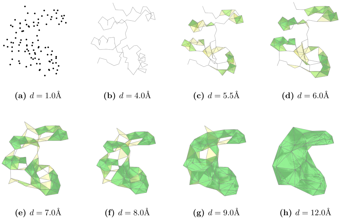
Figura 20: Evolução geométrica do complexo de Vietoris-Rips ao longo da filtração, aplicada sobre uma amostra representativa de 100 carbonos-alfa da estrutura proteica 1OMP. Observa-se a formação progressiva de símplexos de dimensões superiores até a consolidação da topologia global da proteína. As faces de 3-Símplexos são mostradas em verde, os 2-Símplexos em amarelo, os 1-Símplexos como linhas e os 0-Símplexos como pontos.
