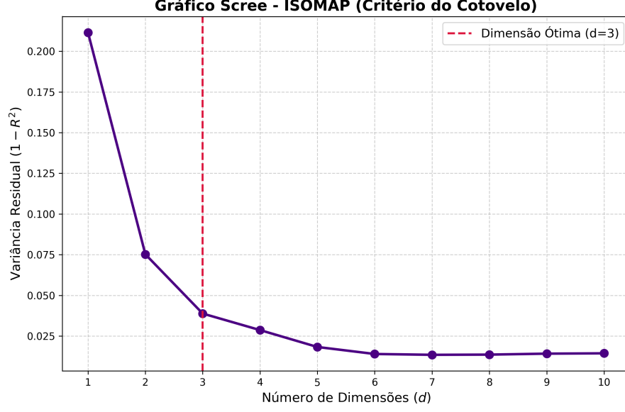
Figura 12: Redução de dimensão via Isomap para a estrutura 1OMP. A flexão abrupta no parâmetro d = 3 indica a dimensionalidade intrínseca ideal para a representação das flutuações dinâmicas da MBP.
