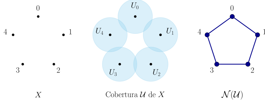
Figura 8: Representação da cobertura \mathcal{U} e do nervo \mathcal{N}(\mathcal{U})
