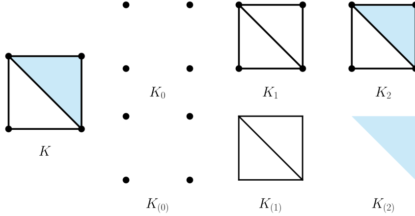
Figura 7: Exemplo do complexo simplicial K_n e o conjunto K_{(n)}
