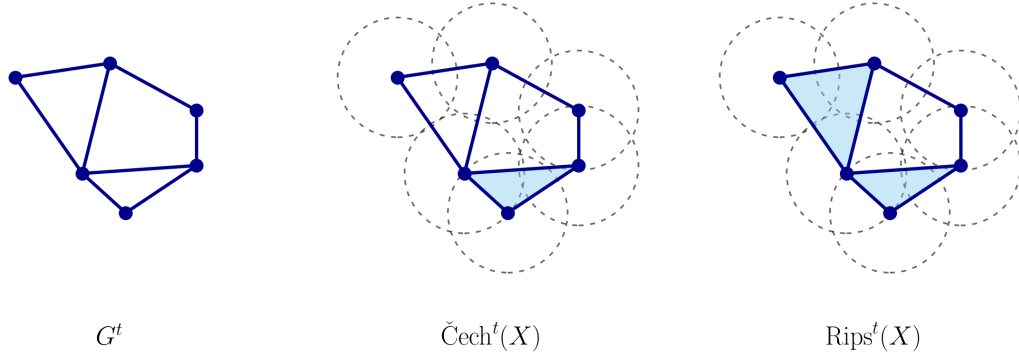
Figura 9: Representação da diferença entre o grafo G^t , o complexo de Čech e o de Rips. Note que o complexo de Čech só possui 1 simplexo de dimensão 2, pois só há uma interseção entre 3 bolas, já o complexo de Rips, há 2 simplexos de dimensão 2, pois basta que as bolas possuam interseções dois a dois.
